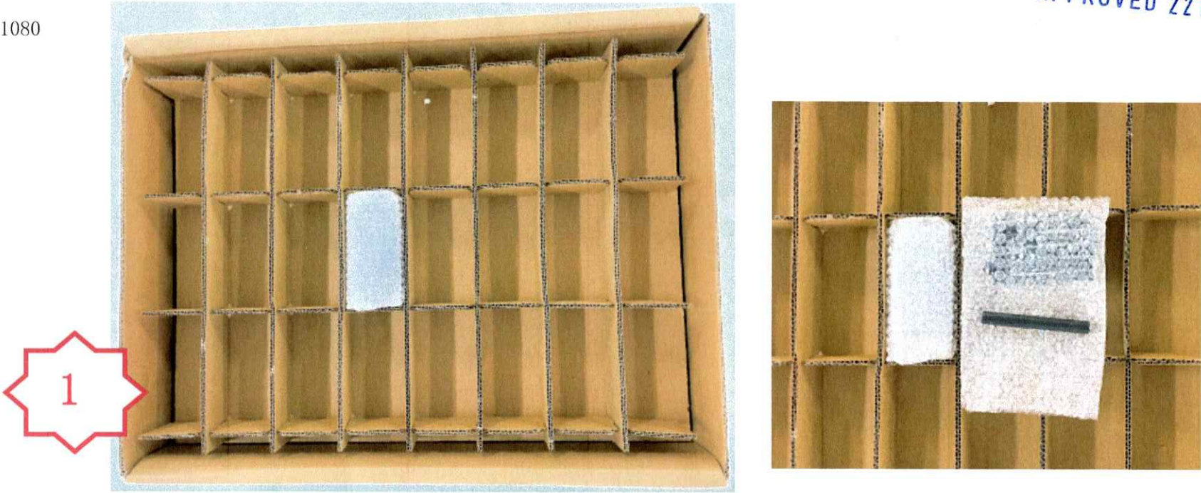
图一，每 5 个组件用一个小气泡袋装，每格 3 袋，每格 15pcs，每层 24 格，每层 360pcs，共 3 层，满箱 1080pcs
